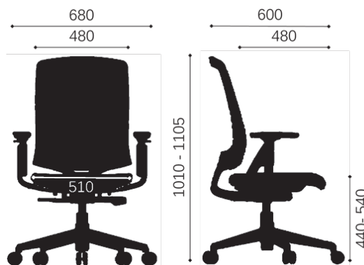
SS.MIR.AP – Armchair
